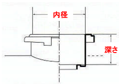
現車フィラーネック(つめ式)
